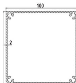
Standard Serie Pillar - 2,465kg / m 100mm x 100mm
