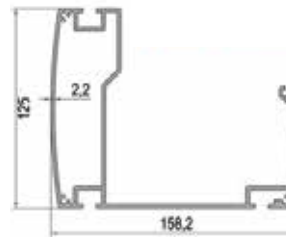
Standard Serie Front Gutter - 3,916 kg / m 158mm x 125mm
