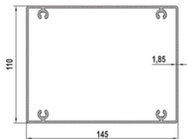
Outstanding Serie Pillar - 3,044kg / m 110mm x 145mm
